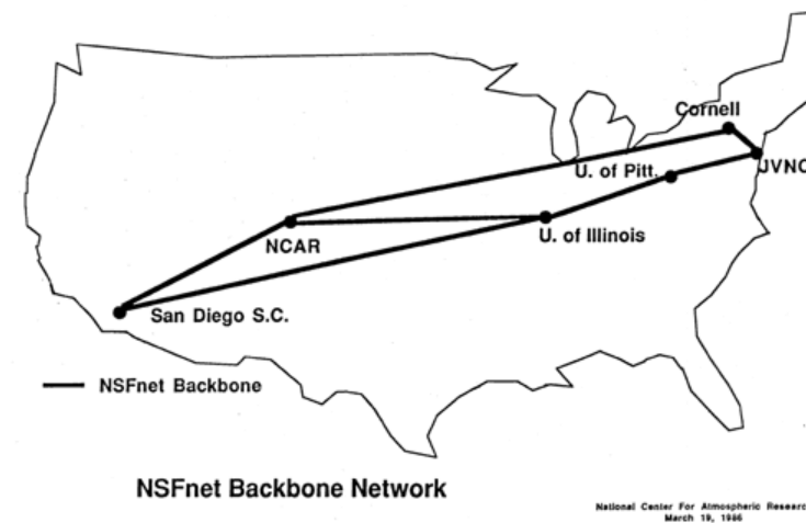
NSFNET Backbone 1986
